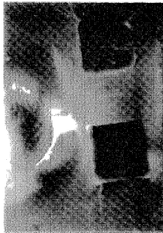
شكل ( ١٥ ) حالات مختلفة على عملة معدنية ( يمين أعلى ) وصليب وطرف اصبع أمامه قطعتان معدنيتان ممغنطتان ( يمين تحت ) ثم قطعة حديد ممغنطة ( يسار تحت ) .. لاحظ اختلاف الهالات الناتجة من تفرع الشحنات على الفيلام الملون .
